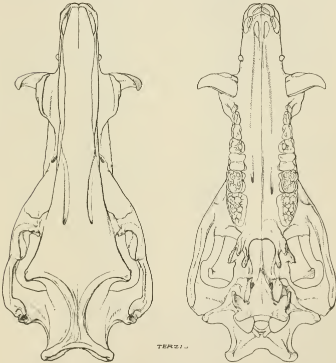
FIG. 199. Sus scrofa . × 1.
