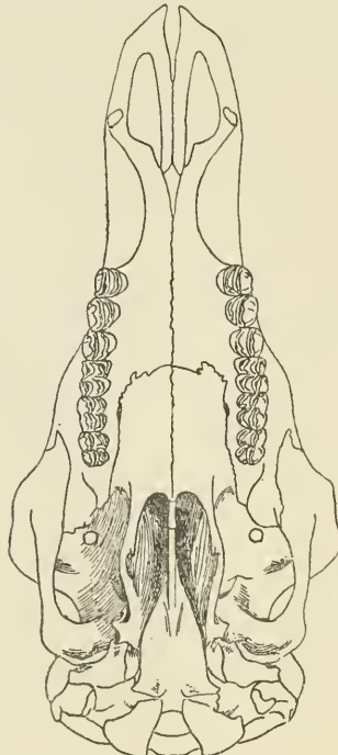
FIG. 210. Rangifer tarandus . × 4.
