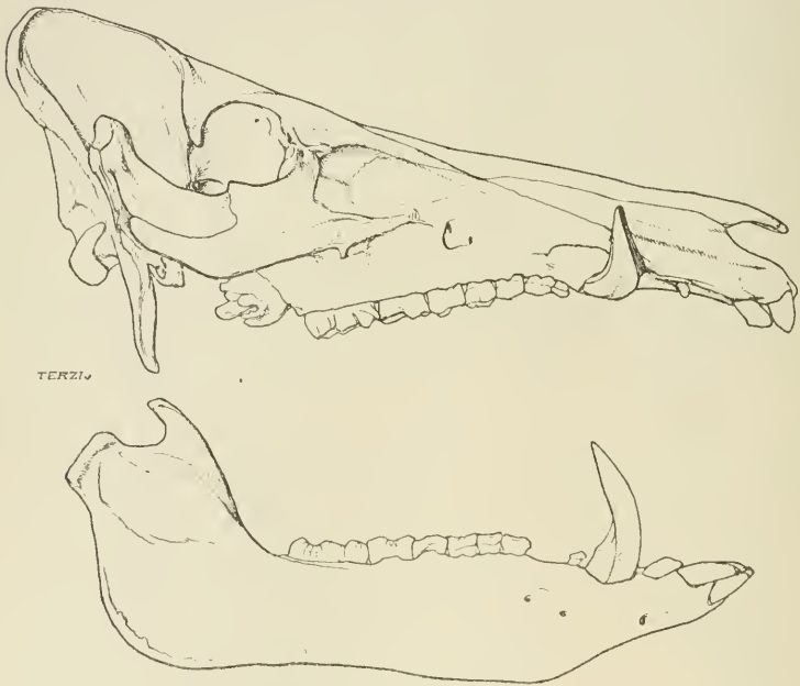
FIG. 200. Sus scrofa. × 4.
