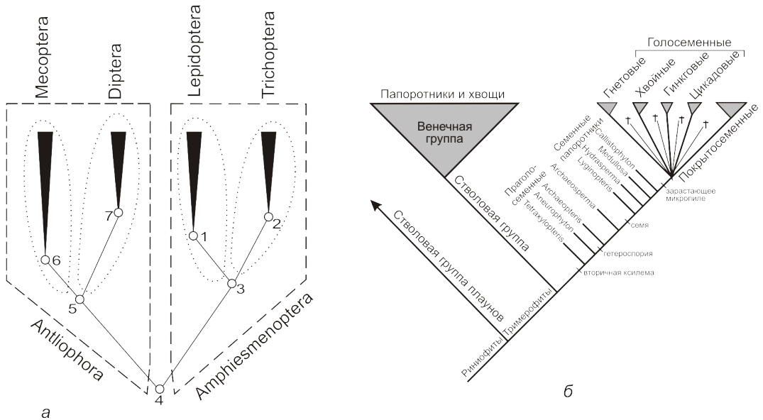
Рис. 13.5. Венечные и стволовые группы. а. Схема филогенетических связей четырех отрядов насекомых (по: Hennig, 1981, fig. 7, p.30, с изменениями); цифрами обозначены предковые формы; б. Упрощенная кладограмма связей сосудистых растений (по: Kenrick, Crane, 1997; Pryer et al., 2004).
