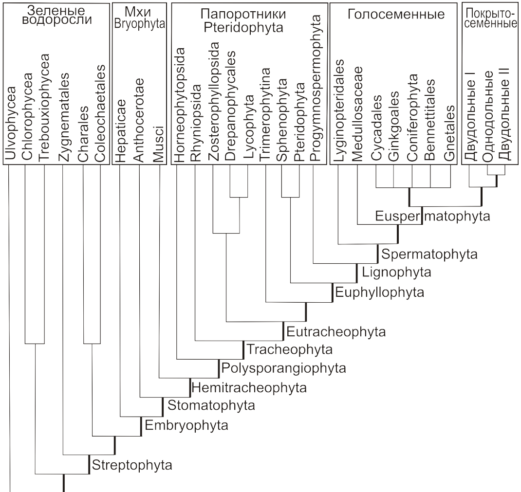
Рис. 13.2. Схема филогенетических связей основных групп растений (по: Kenrick, Crane, 1997; Niklas, 1997 и другим авторам).
