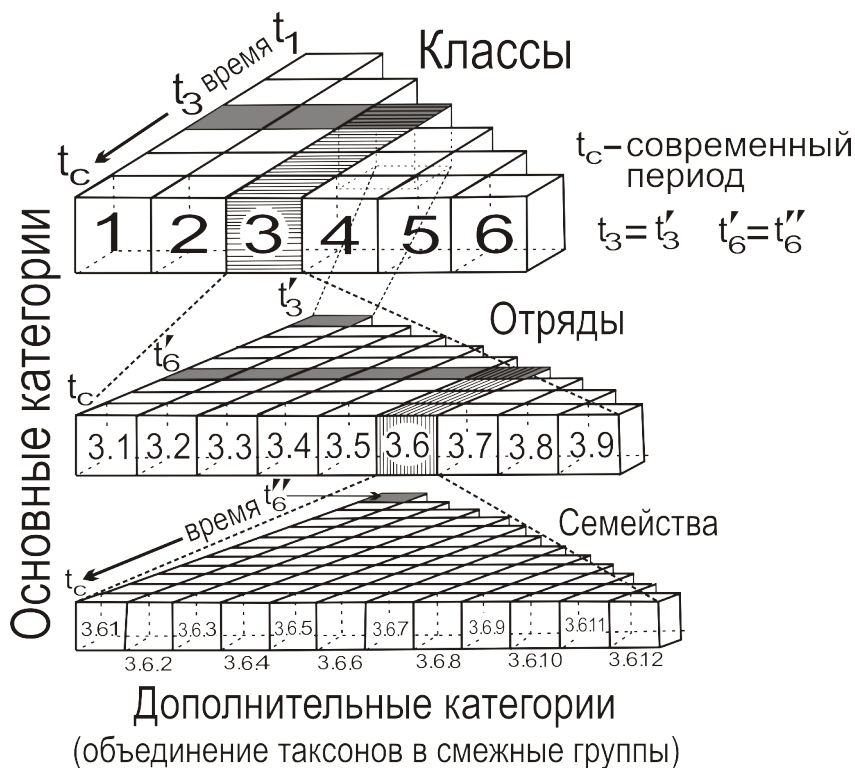
Рис. 2. Идеализированная структура связей основных (классы, отряды и семейства) и дополнительных таксономических категорий (пояснения в тексте). цифрами 1–6, 3.1–3.9, 3.6.1–3.6.12 обозначены классы, отряды и семейства соответственно; t — временные интервалы.
