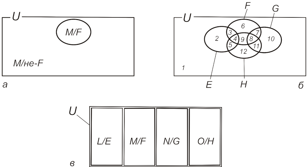
Рис. 11.1. Выделение групп по заданным свойствам. U — исследуемое множество; E , F , G , H — свойства; цифрами и символами вида M/F обозначены различные подмножества U (см. также текст).
