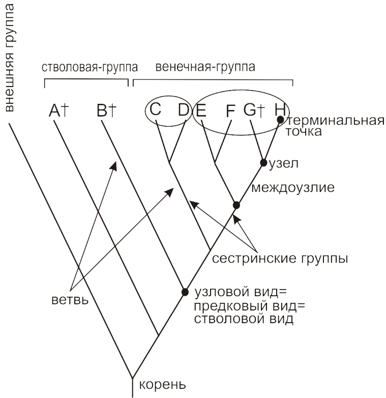
Рис. 12.2. Филогенетическое дерево и его элементы и части. Буквами обозначены терминальные таксоны; крестиком помечены вымершие таксоны.
