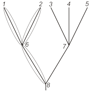
Рис. 1.10. Модель вида в рамках принципа дихотомии. Цифрами обозначены виды.
