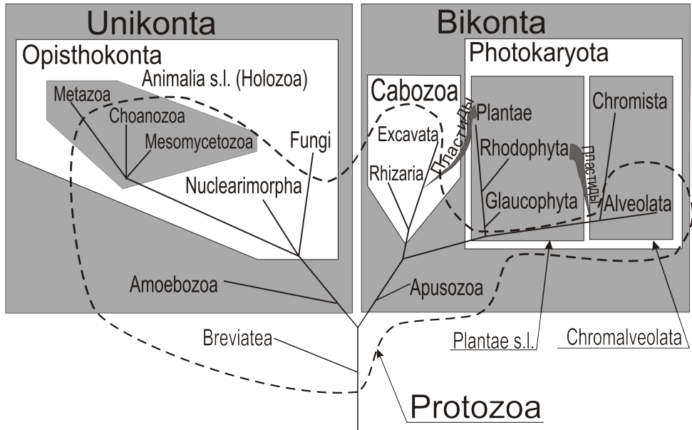
Рис. 10.10. Кладограмма связей и классификация эукариотических организмов (по: Cavalier-Smith, 2002в, 2004, с изменениями).
