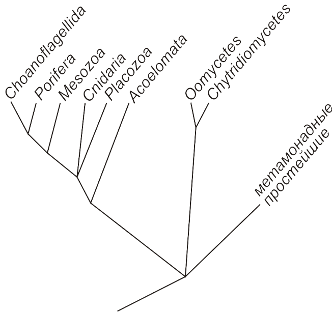
Рис. 12.11. Положение и филогенетические связи низших животных (хоанофлагелляты и нецеломические животные). По: Lipscomb, 1985, fig. 1.
