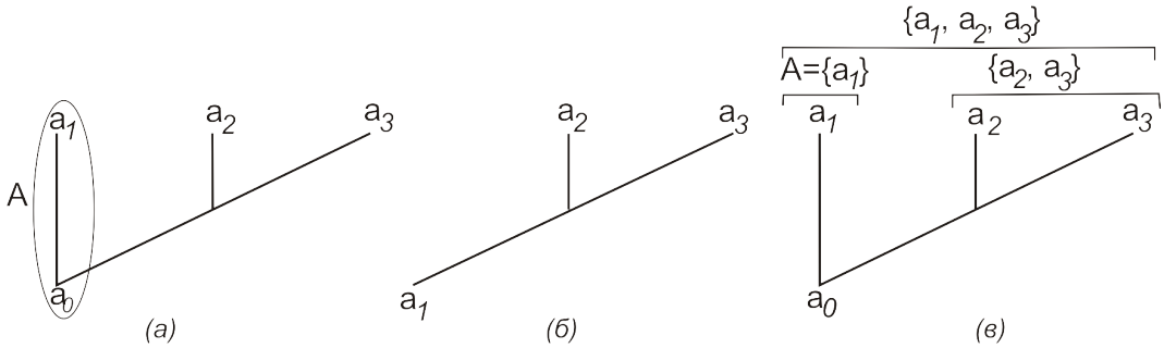
Рис. 13.9. Парадокс Платника. a_1 — виды, фигурными скобками выделены группы (пояснения в тексте).
