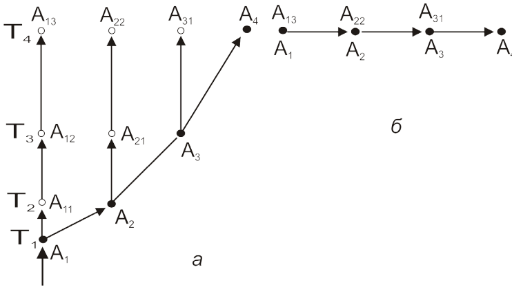
Рис. 14.5. Экологические ограничения и асимметрия кладограмм. Генеалогическое (а) и филогенетическое (б) представление эволюции (пояснения в тексте). A_i — таксоны; t_i — время.
