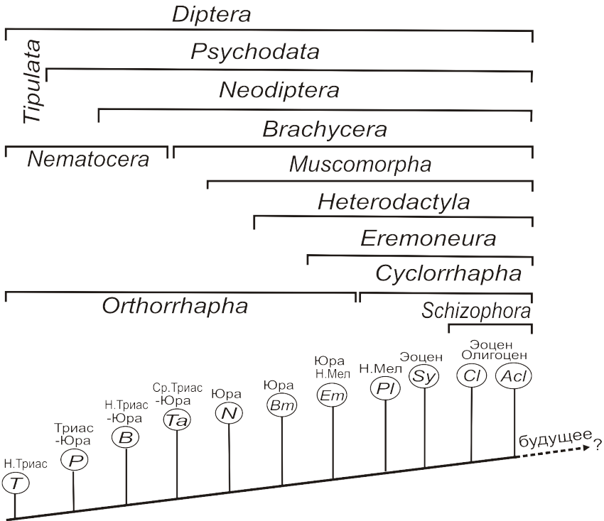
Рис. 1.2. Кладограмма двукрылых насекомых с указанием приближенных оценок времени появления терминальных таксонов. Т — Tipuloidea; Ps — Psychodoidea; B — Bibionoidea; Ta — Tabanoidea; N — Nemestrinoidea; Bm — Bombylioidea; Em — Empidoidea; Pl — Platypzoidea; Sy — Syrphoidea; Cl — Calyprata; AcI — Acalyprata.
