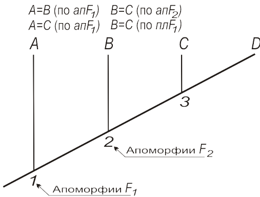
Рис. 11.7. Кладogramма четырех таксонов A, B, C, D. апF — синапоморфный комплекс признаков F; плF — симплезиоморфный комплекс признаков F (пояснения в тексте).
