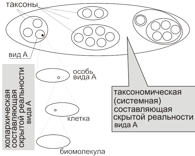
Рис. 6.1. Вертикальная и горизонтальная составляющие «скрытой реальности». Горизонтальная определяется таксономическим положением организма, вертикальная — его связями с холонами высших и низших уровней.
