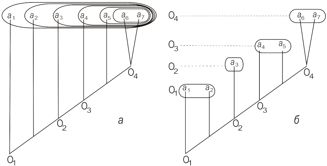
Рис. 12.15. Вертикальная классификация (а) и горизонтальные классификации (б), определяемые относительно точек ветвления o_i . a_i — терминальные таксоны.
