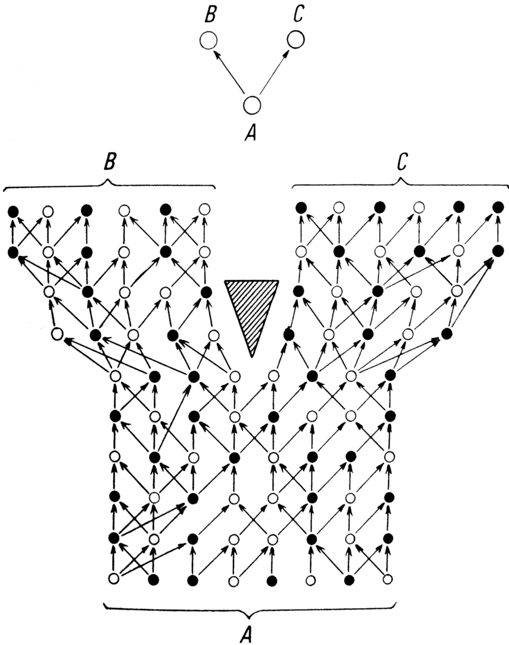
Рис. 9.6. Схема разделения материнского вида А на два дочерних вида В и С (по: Hennig, 1966, fig. 4).
