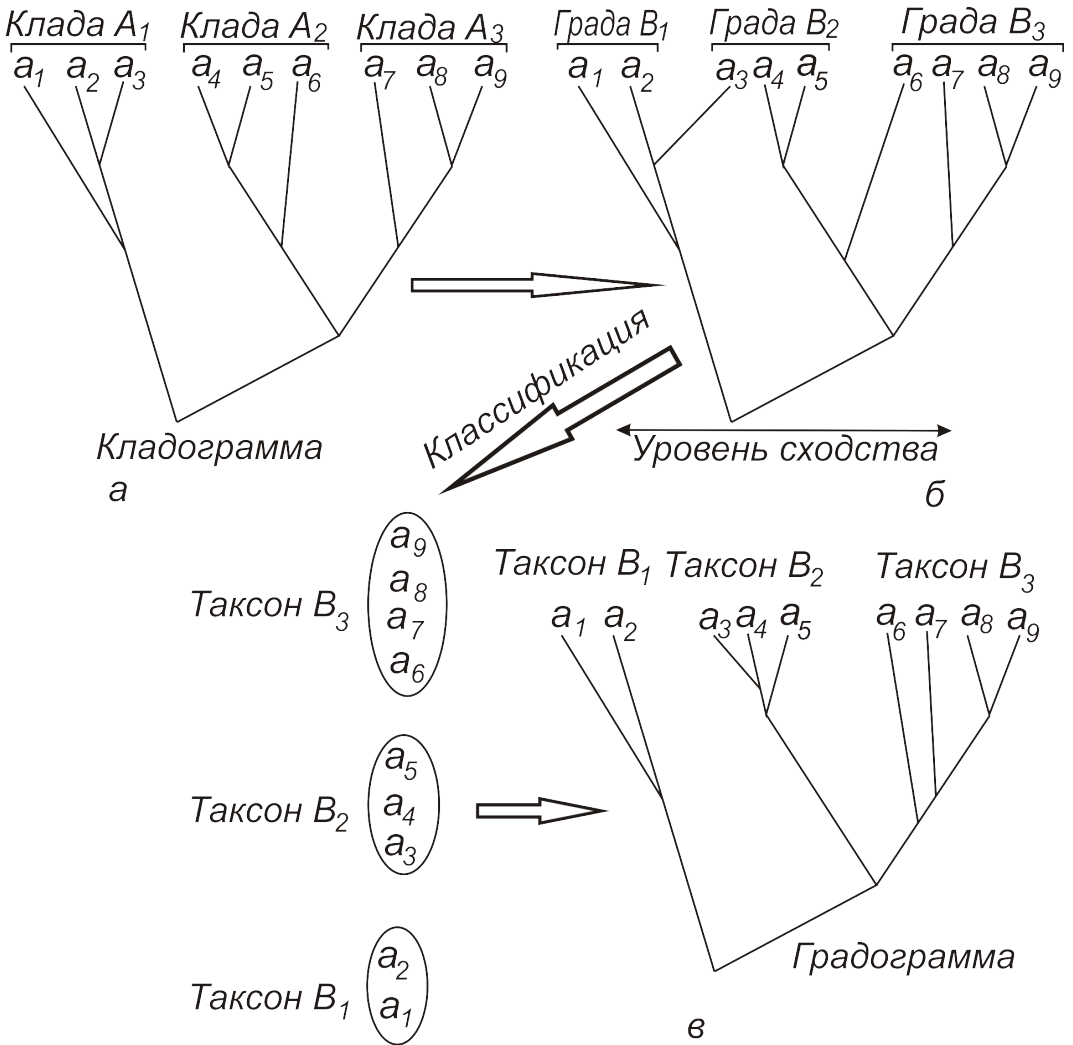
Рис. 12.7. Соотношение между кладограммами, кладами, градограммами и градами. а 1 — терминальные таксоны (пояснения в тексте).
