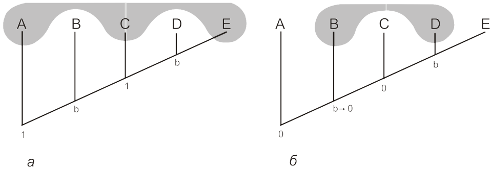
Рис. 13.18. Альтернативные способы разбиения кладограммы (пояснения в тексте).
