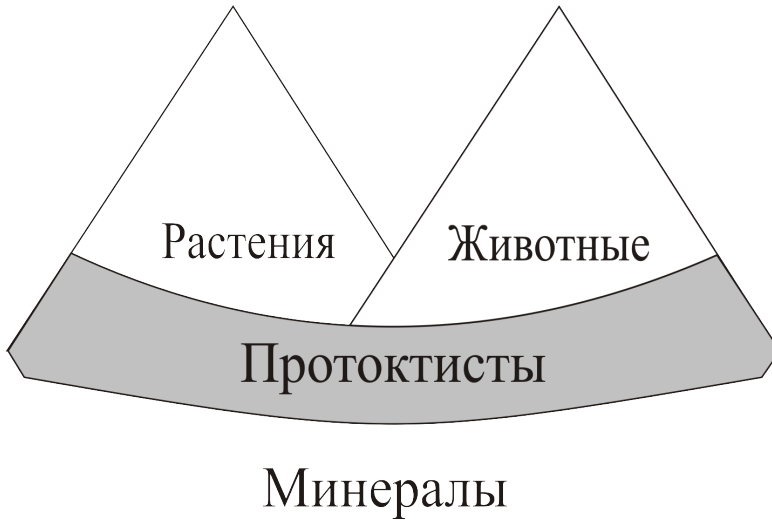
Рис. 10.2. Четырехцарственная система натуралей (Hogg, 1860).
