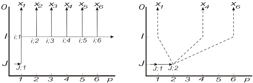
Рис. 14.4. Фрагменты онтогенетических траекторий в установившемся (а) и измененном (б) режимах. o_i , o_j — последовательные онтогенетические уровни; p_i — внутриуровневая последовательность онтогенетических событий, отражающая процессы анагенетического накопления инноваций; x_p — таксоны, для видов которых приведены фрагменты онтогенетических траекторий.
