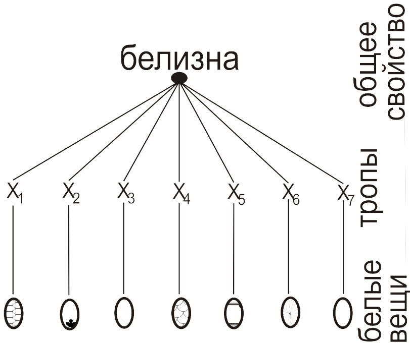
Рис. 2.4. Свойство близны, опосредуемое через тропы (объяснение в тексте).
