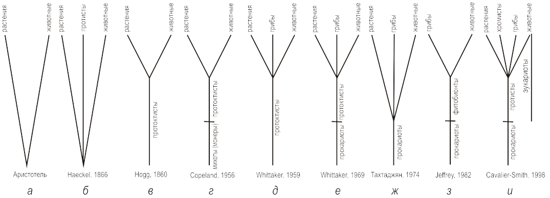
Рис. 10.1. Схемы горизонтального и вертикального деления древа организмов по разным авторам.
