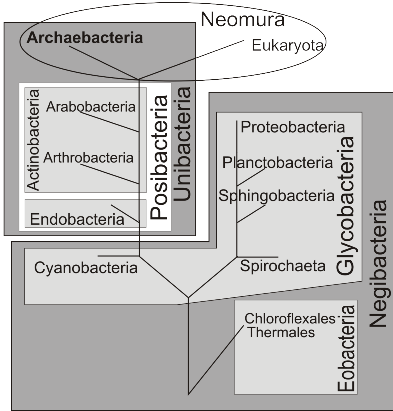
Рис. 10.8. Кладограмма связей и классификация организмов, рассматривающая в качестве исходной формы двуplenочного предка (по: Cavalier-Smith, 2002a, fig. 2, p.20; из Шаталкин, 2004б).
