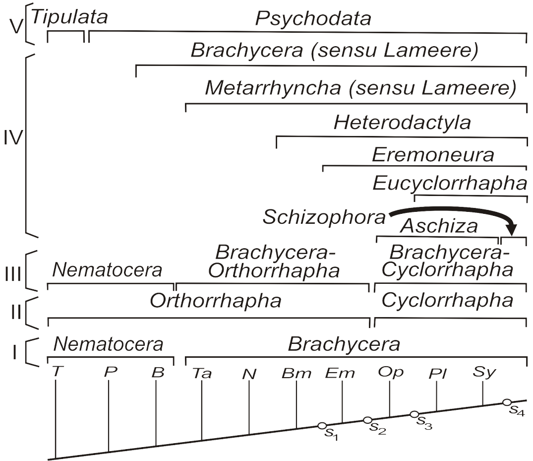
Рис. 14.1. Схема кладограммических связей двукрылых насекомых с выделенными на ней небазисными группами. s_1 - s_4 — тестируемые синапоморфии внутри области, разделяющей прямошовных и круглошовных мух; I-V — различные схемы деления двукрылых на небазисные группы: I — по Macquart, II — по Brauer, III — по Osten-Sacken, IV — по Lameere, V — по Steyskal; T — Tipuloidea; P — Psychodoidea; B — Bibionoidea; Ta — Tabanoidea; N — Nemestrinoidea; Bm — Bombylioidea; Em — Empidoidea; Op — Opetiidae; Pl — Platypzoidea; Sy — Syrphoidea (терминальные таксоны концевой участка дерева, отвечающие группе Schizophora не указаны).
