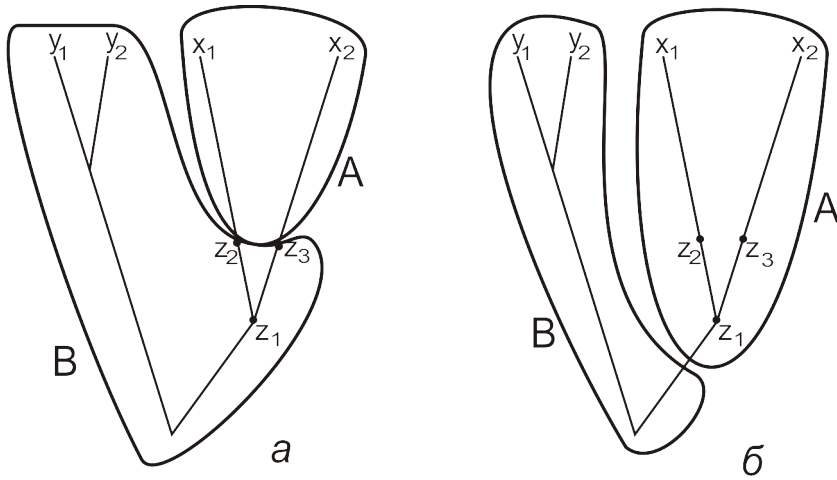
Рис. 13.14. Полифилия (а) и монофилия (б) групп в зависимости от способа их выделения. А, В — надвидовые таксоны; x_i, y_i — рецентные виды, z_i — предковые формы.
