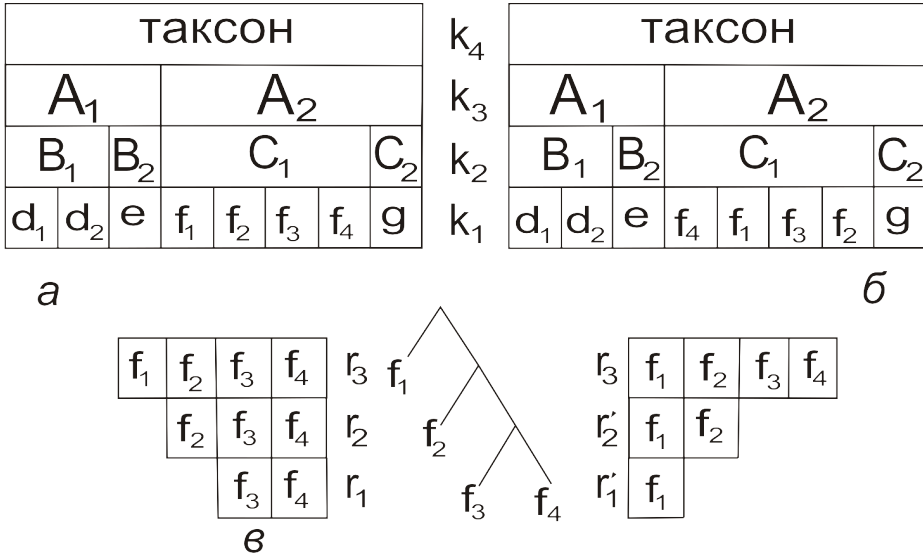
Рис. 1.1. Классификация и систематизация (объяснение в тексте). A 1 , B 1 , C 1 , d 1 , e, f 1 , g — таксоны; k 1 , r 1 — таксономические категории.
