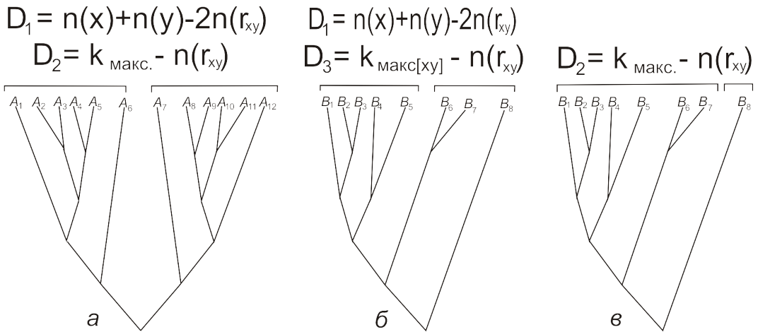
Рис. 11.8. Классификации, основанные на исчислении вертикальных (кладограммы а, в) и горизонтальных (кладограмма б) связей. A_i, B_i — терминальные таксоны.
