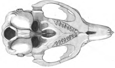
Fig. 2. Canis lupus
