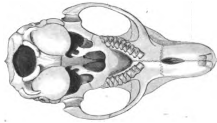
Fig. 4. Canis lupus
