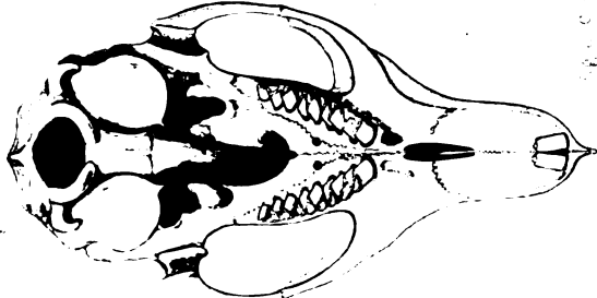
Fig. 5. Canis lupus
